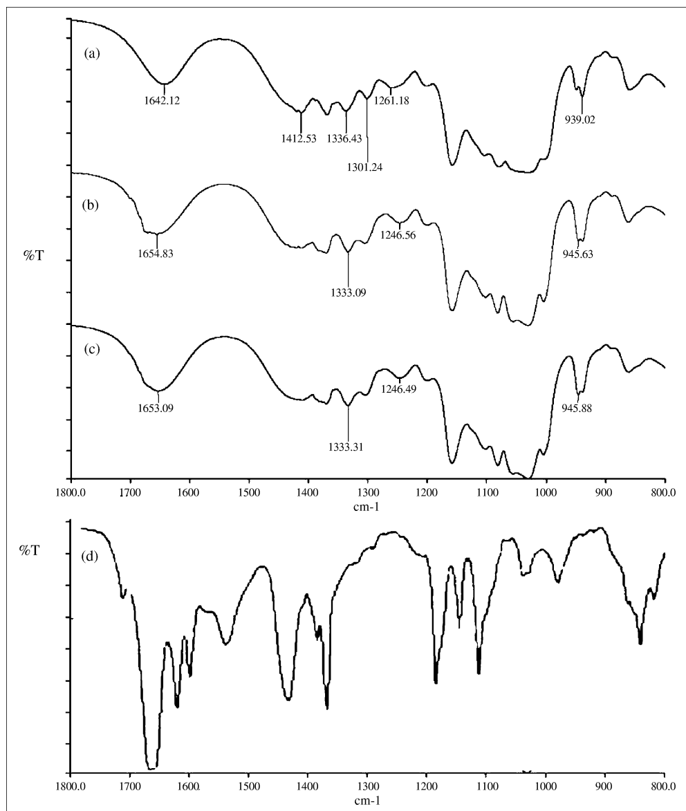
Fig. 1: IR spectra of (a) \beta -CD; (b) \beta CD-LVO-SD, (c) \beta CD-LVO-PR, and (d) citral
