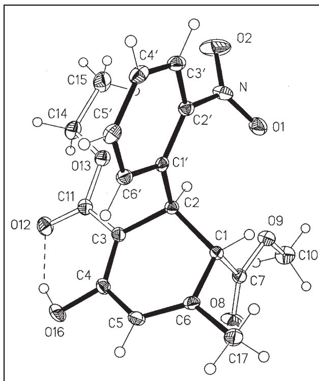
Abb. 3: Röntgenkristallstruktur von 4bC . Ellipsoide entsprechen 30%iger Aufenthaltswahrscheinlichkeit
