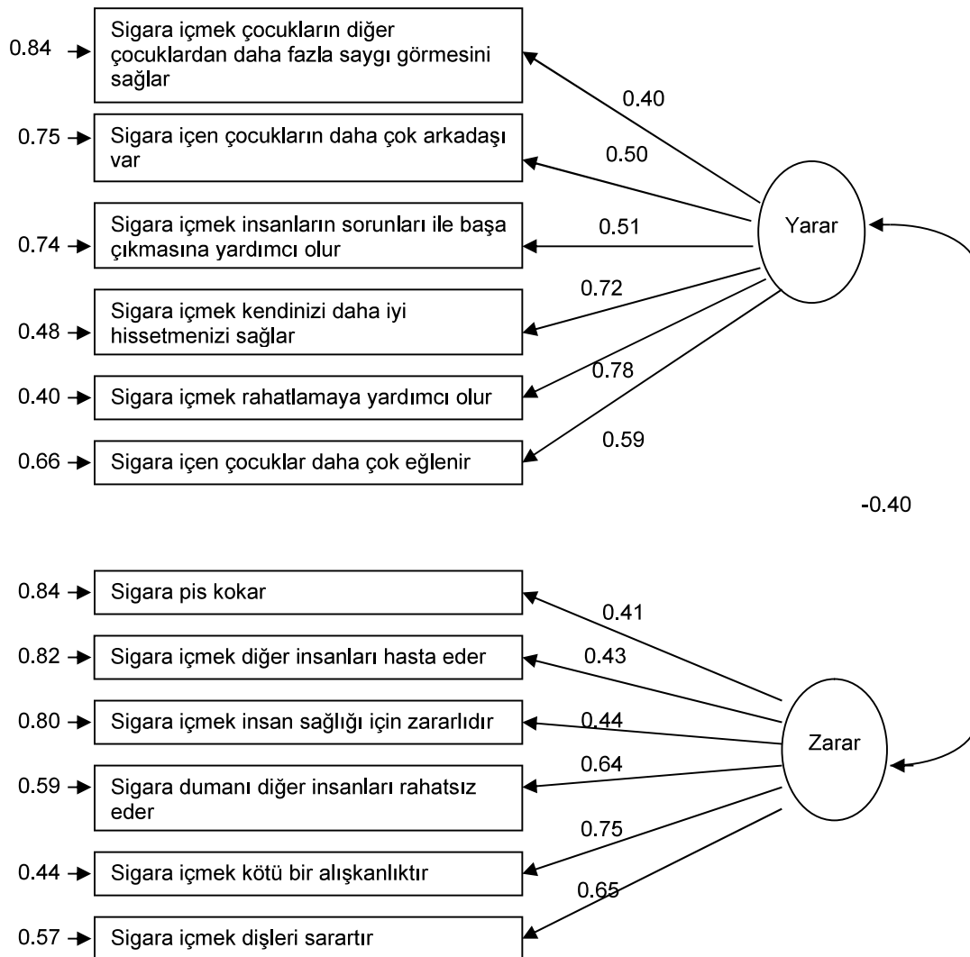
Şekil 1. Karar Denge Ölçeğinin doğrulayıcı faktör analiz modeli
